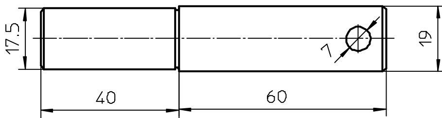
Drehteil
