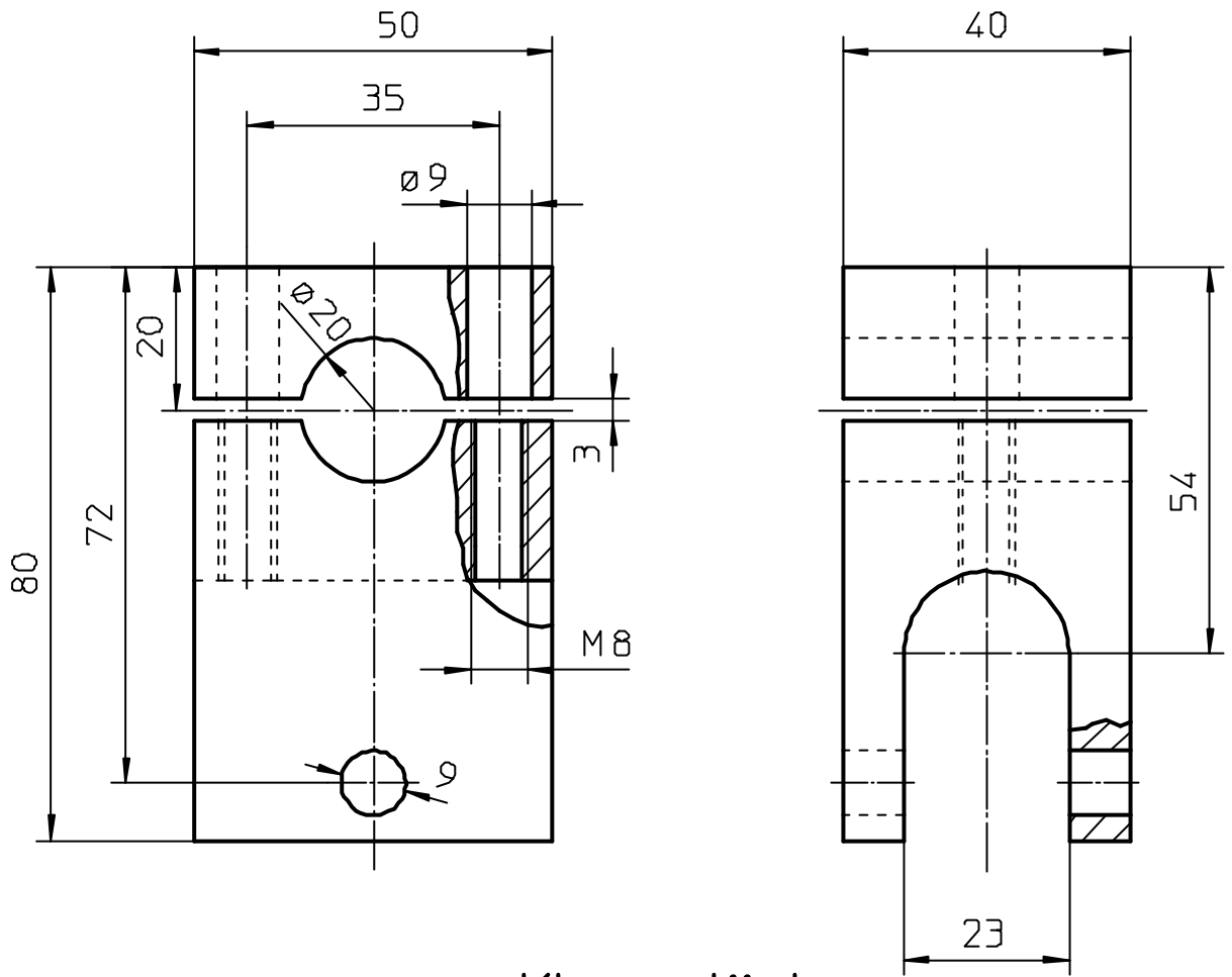
Klemmstück
